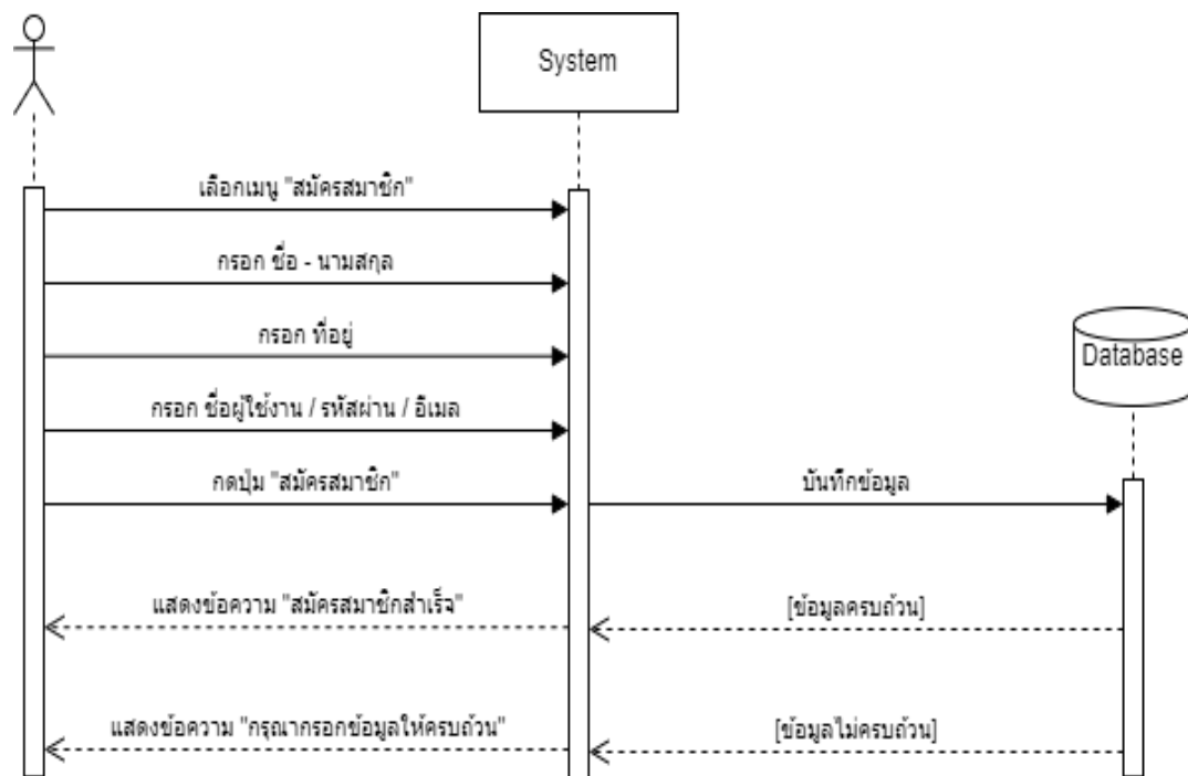
ตัวอย่าง Sequence Diagram
